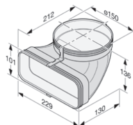
Kompakt adapter DFK-AK 90
