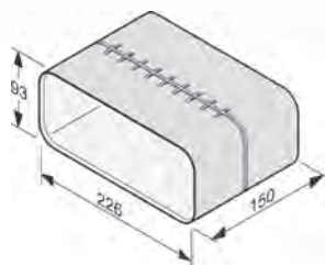
Forlængerstykke DFK-L
