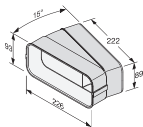
Rørbøjning 15° horizontal DFK-BH 15
