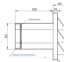
Murkasse fladkanal DFK-M
