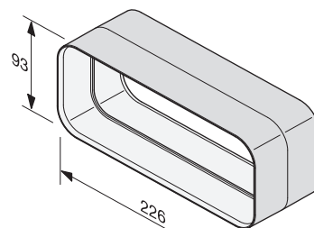
Samlestykke DFK-V
