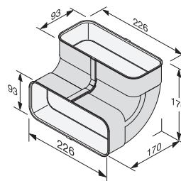
Rørbøjning 90° vertikal DFK-BV 90
