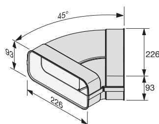
Rørbøjning 45° horizontal DFK-BH 45
