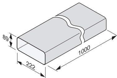
Lige stykke DFK-R 1000
